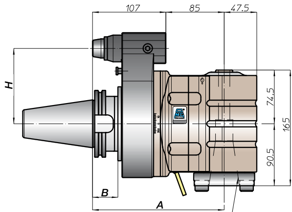
Cono 40 DIN2079
