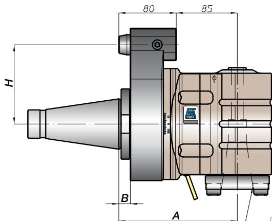
Cono 40 DIN2079
