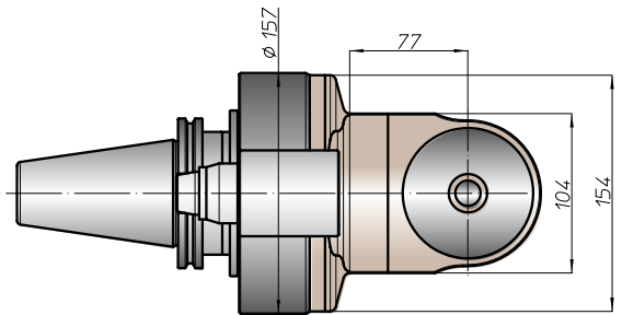
Cono 40 DIN2079
